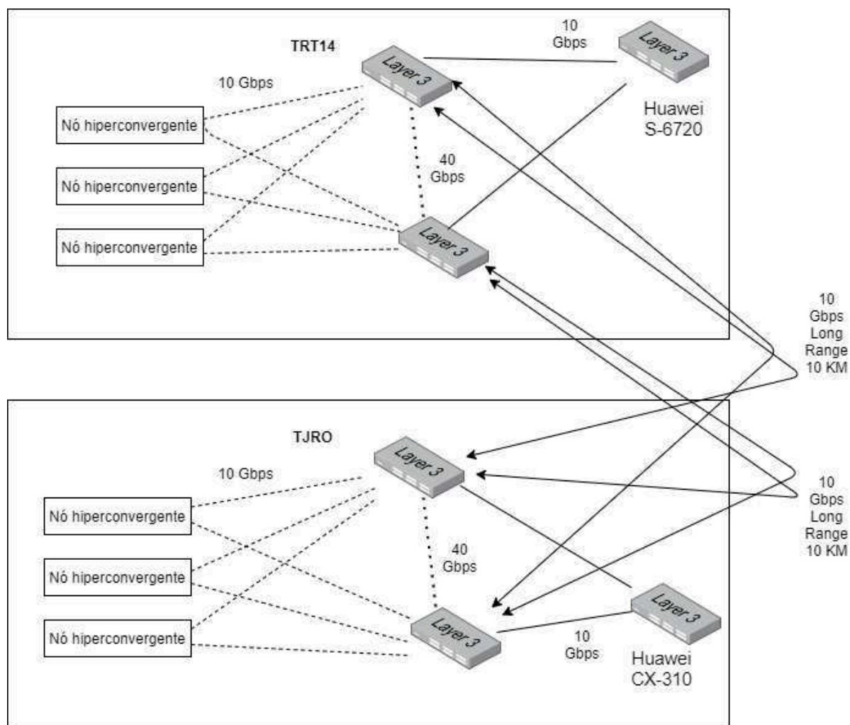
Figura 4: Topologia de rede da solução
